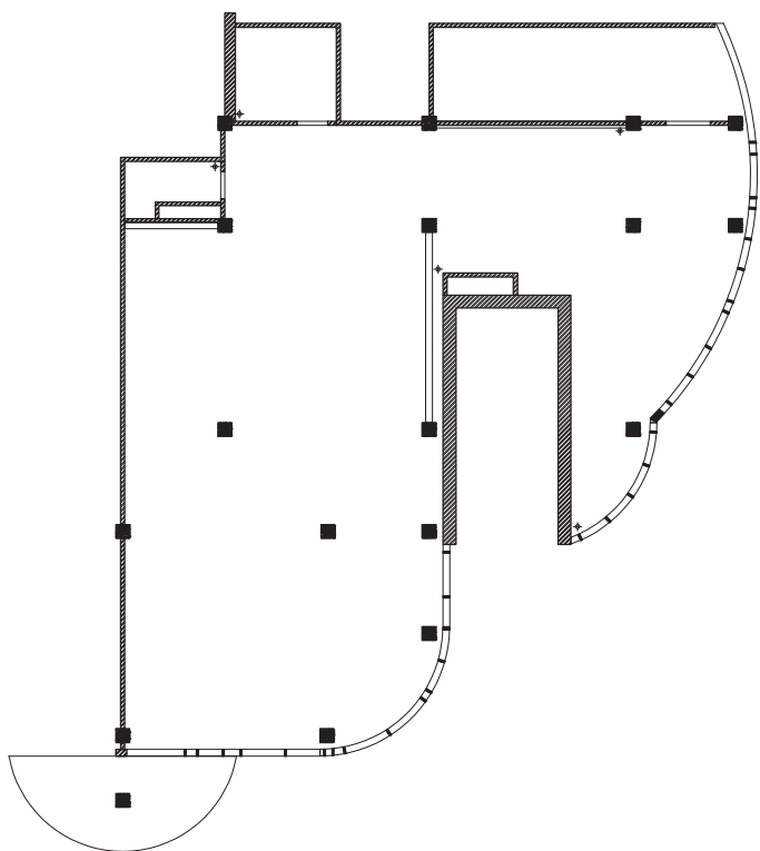
План до реконструкции
